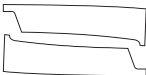
2. Gabarits pour enjoliveur de seuil de porte avant
